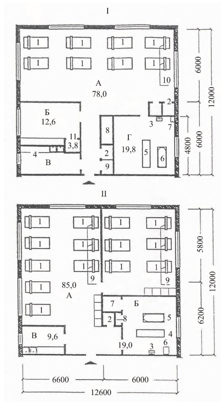
I – планировочная схема жилых комнат жилой ячейки типа 1в для лежачих детей с сохранным интеллектом
